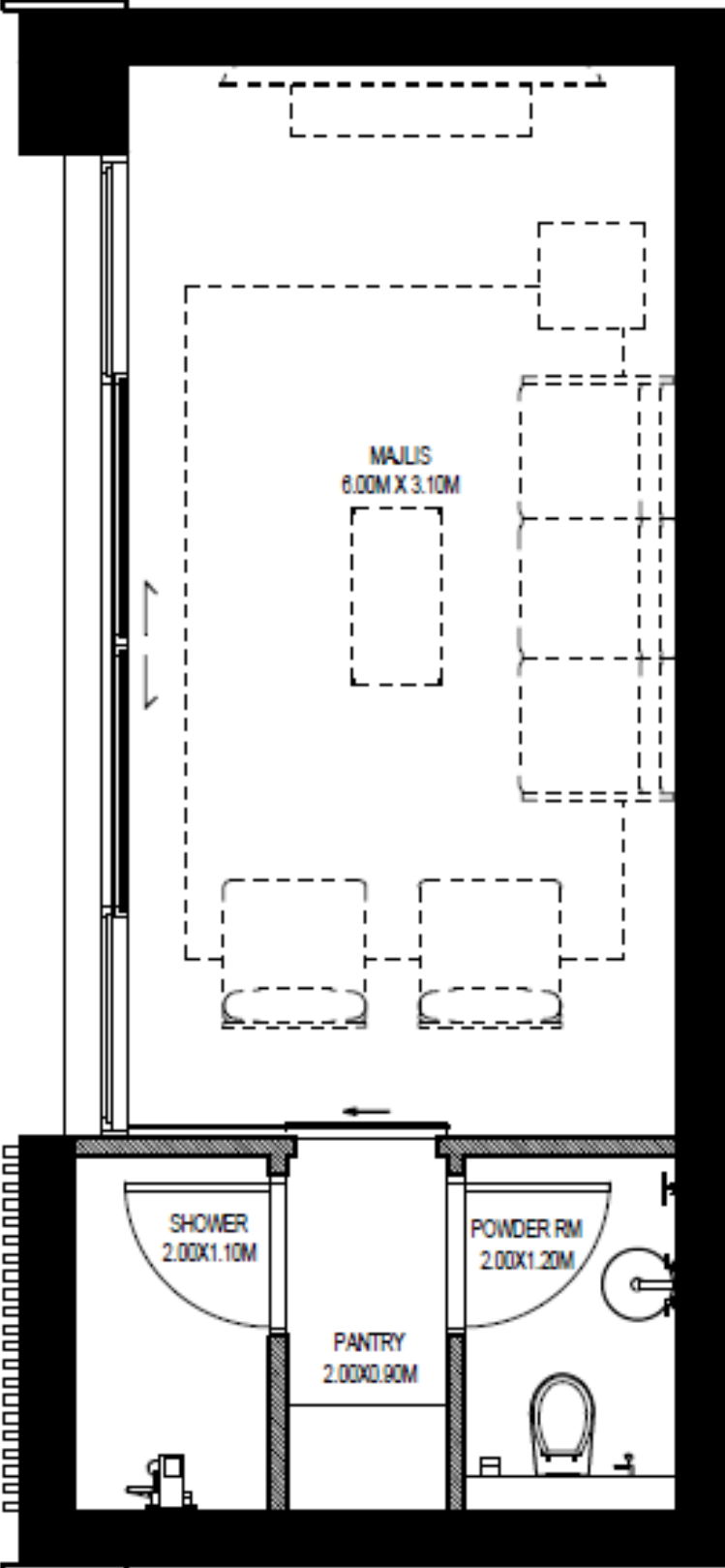
MAJLIS LAYOUT
